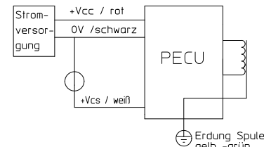
Schaltplan für Signal 0-10V Abb.2a
