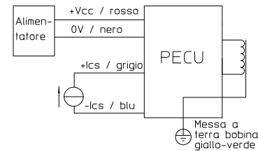
Schema di collegamento per segnale di controllo 4-20mA fig.2b
