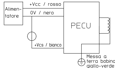
Schema di collegamento per segnale di controllo 0-10V fig.2a
