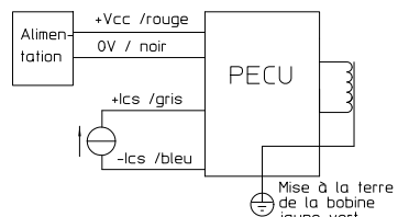
Schéma de câblage pour signal de commande 4-20mA fig.2b
