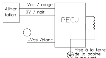
Schéma de câblage pour signal de commande 0-10V fig.2a
