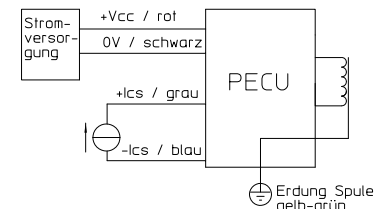
Schaltplan für Signal 4-20mA Abb.2b
